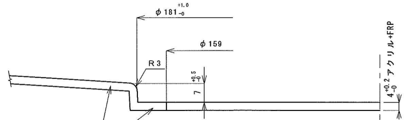
B断面図 縮尺1:1 排水口部
