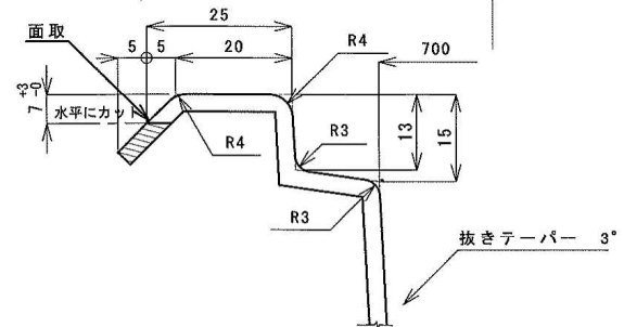
A断面図 縮尺1:1
